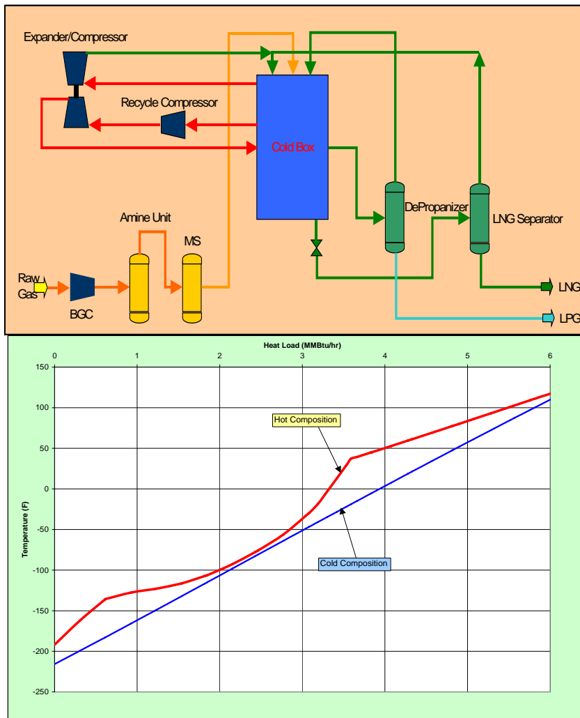
图-2：KRYOPAK EXP 工艺简图及 Q/T 图
